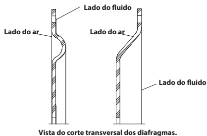
Vista do corte transversal dos diafragmas.
